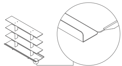
Profile for 400mm base Perfil para base de 400mm
