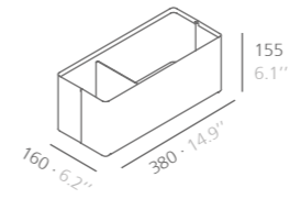
Box Cajón
