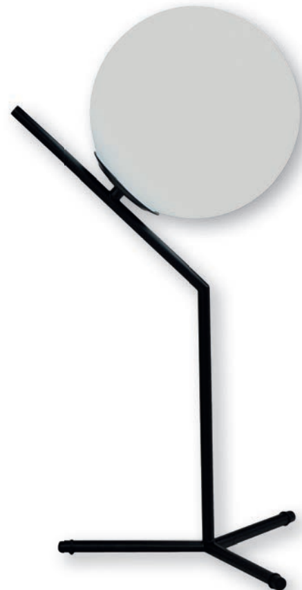
Lámpara de mesa 825-C-N Estructura metal, acabado negro Globo de vidrio soplado blanco 28*53 cm. Casquillo E14
