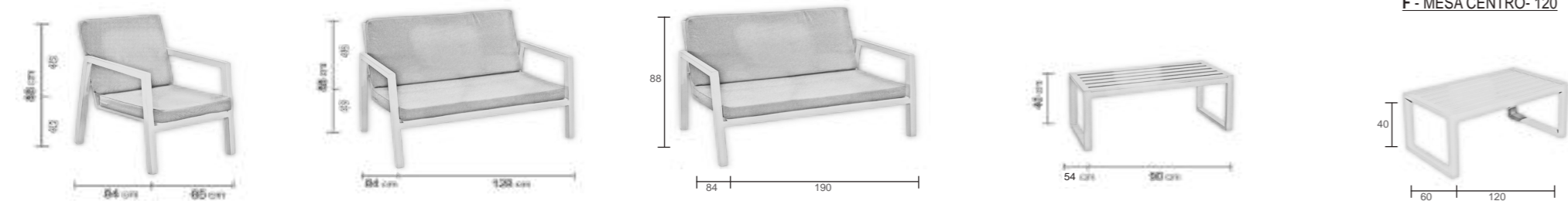
A - ÁGATA-1 B - ÁGATA-2 C - ÁGATA-3 E - MESA CENTRO -90 F - MESA CENTRO- 120
